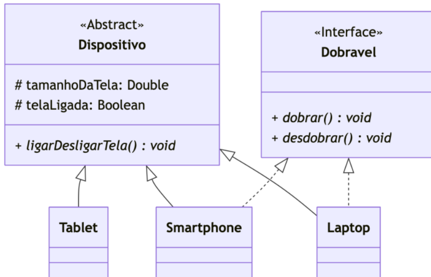
Figura 1: Diagrama de classes dos dispositivos móveis.
